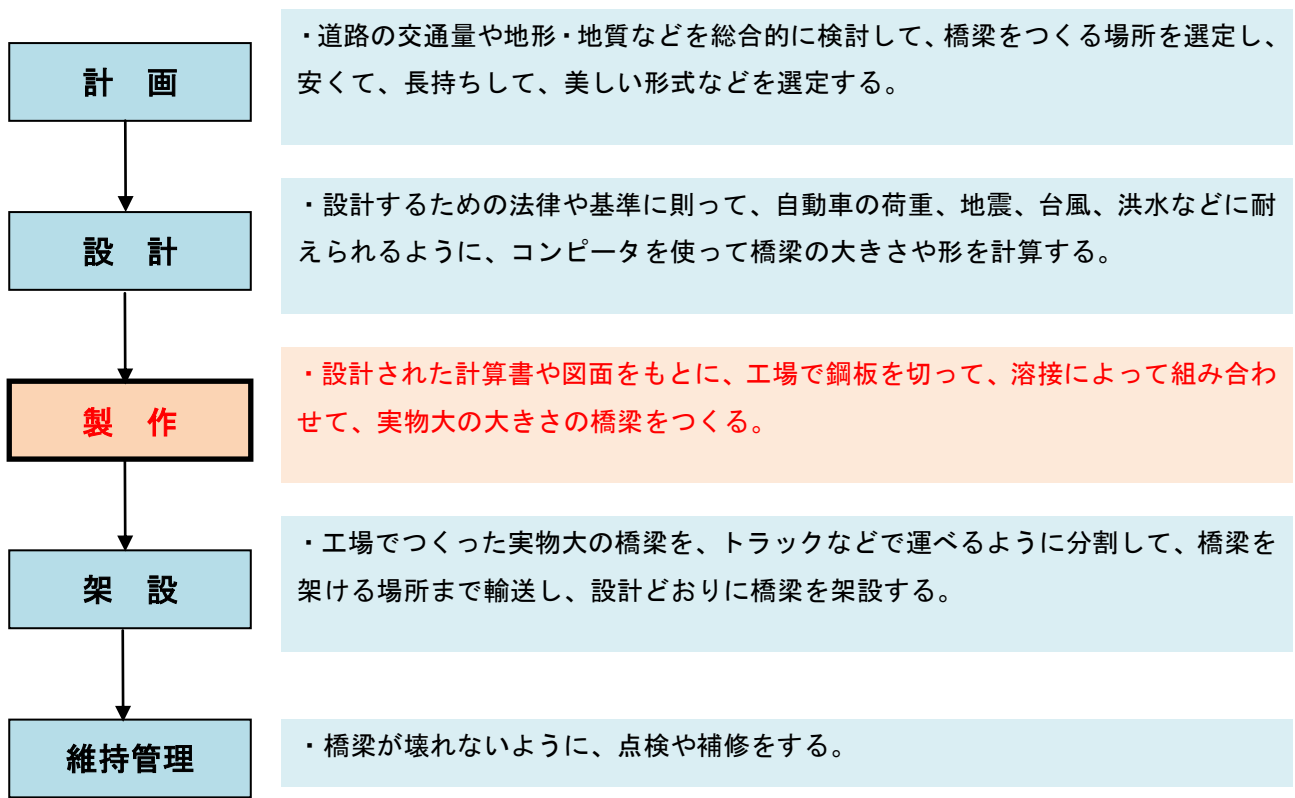
図-1 橋梁の計画から維持管理までの流れ
